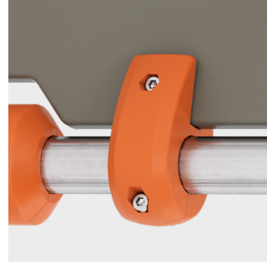
22 СОЕДИНИТЕЛЬ «HDPE-ТРУБА» Стеклонаполненный полиамид Предназначен для крепления HDPE-пластика (15 мм) к трубе ДУ25.
